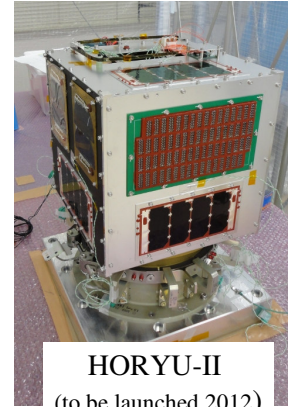
HORYU-I
